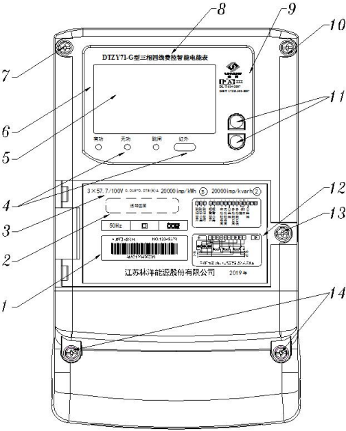
图2 外形图
