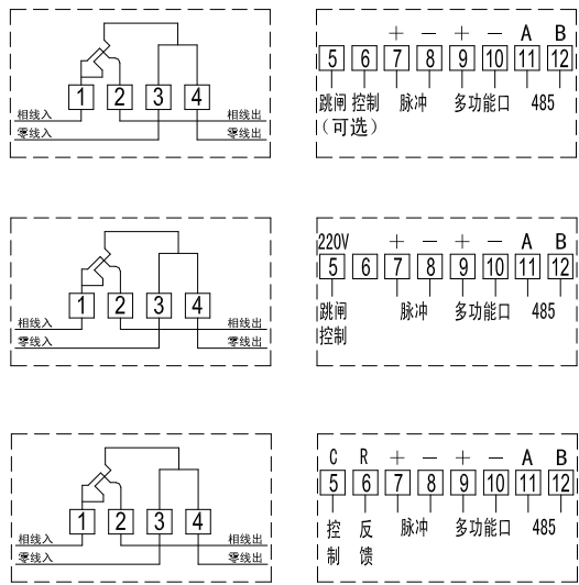
图 3：直接接入式
