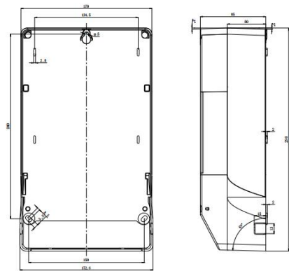
图3 安装尺寸
