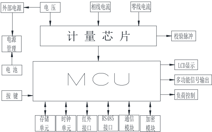
图 1：基本工作原理框图
