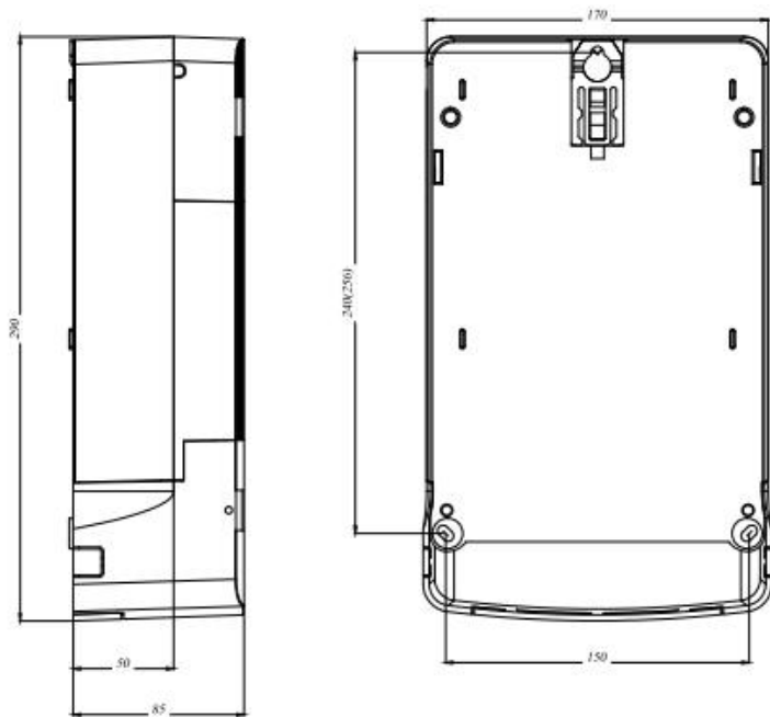
图4 安装尺寸
