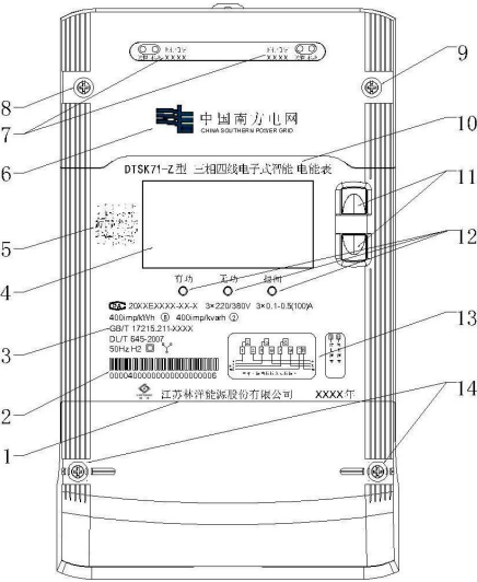
图3 外形图
