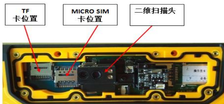
图 2-1 卡座位置示意图
