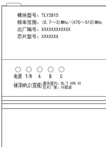
图 2-1 集中器模块外观示意图
